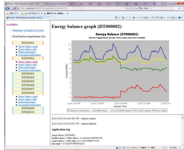
図 4 盗電検知システム画面
