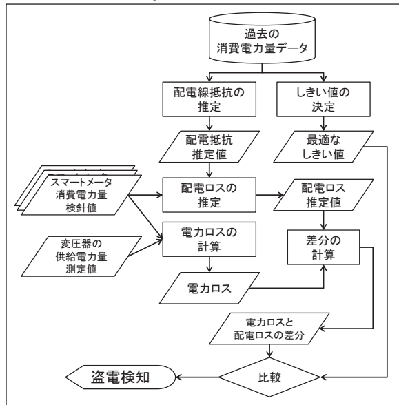
図 3 盗電検知フロー
